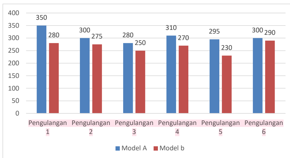
Gambar 4.1. Grafik Hasil Pengukuran Berat Bioarang Kulit Kakao dari Pengolahan Model Alat Pirolisis Kulit Kakao
