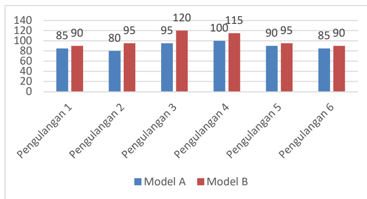
Gambar 4.2. Grafik Hasil Pengukuran Volume Asap Cair Kulit Kakao dari Pengolahan Model Alat Pirolisis Kulit Kakao
