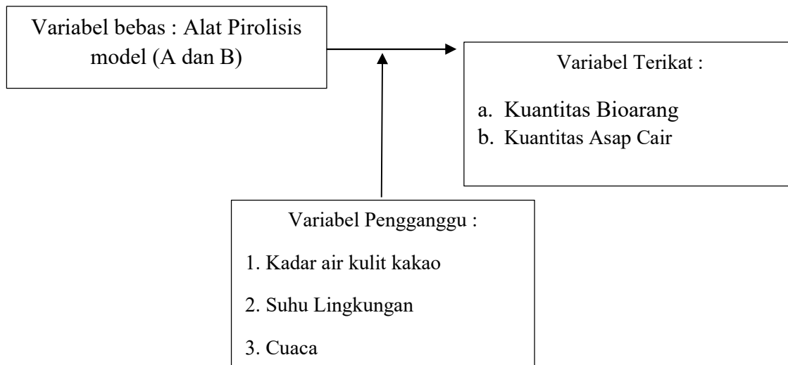
Gambar 3.1 Hubungan antar Variabel
